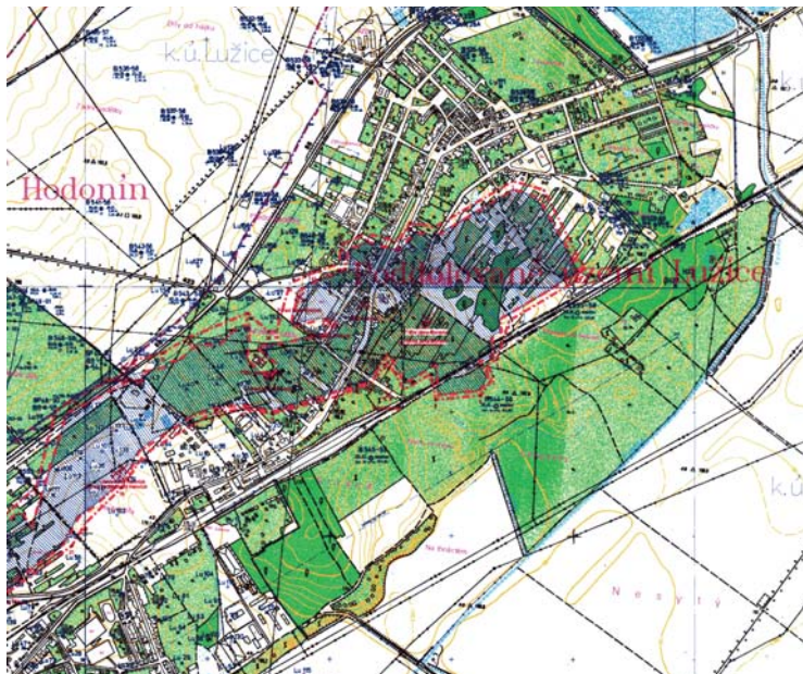
Rozsah poddolování, k. ú. Lužice u Hodonína
